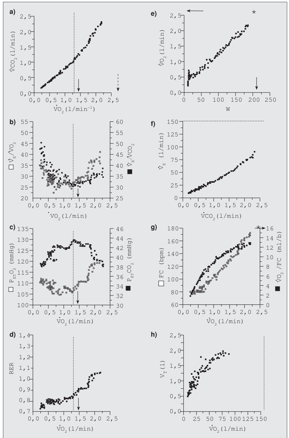
Fig. 1. Resultado del ejercicio en un sujeto sano sedentario de 42 años. Presentación de los gráficos básicos recomendados para la interpretación de las pruebas de ejercicio cardiopulmonar (PECP). En las gráficas (a-d) de la columna izquierda se indica el \dot{V}O_2 (abscisas) en relación a las variables comúnmente usadas para estimar de manera indirecta el umbral láctico (LT, ver Apéndice). La línea vertical discontinua representa el \dot{V}O_2 en la zona de transición desde ejercicio de moderada a severa intensidad. El LT esperado para un sujeto sano (55% del valor de referencia del \dot{V}O_2 pico) se representa con una pequeña flecha de trazo continuo. El valor de referencia del \dot{V}O_2 pico se indica en el gráfico a) con una flecha de trazo discontinuo. En la columna de la derecha, el gráfico e) indica el \dot{V}O_2 frente a trabajo (vatios). Los valores máximos alcanzados en \dot{V}O_2 y vatios indican la tolerancia al ejercicio del sujeto. Los valores de referencia correspondientes se indican con un asterisco. Los gráficos f) y h) indican la respuesta de la ventilación frente a \dot{V}CO_2 y volumen corriente frente a ventilación. La línea de trazo discontinuo representa la ventilación máxima esperada. La diferencia entre ésta y la ventilación máxima alcanzada por el sujeto es la reserva ventilatoria. Finalmente, el gráfico g) presenta las características de la respuesta hemodinámica (frecuencia cardíaca y pulso de oxígeno) al ejercicio. El valor de referencia de la frecuencia cardíaca máxima se representa por un asterisco y por una flecha el pulso de oxígeno.
